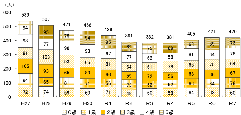
図 2-20 人口の推移
