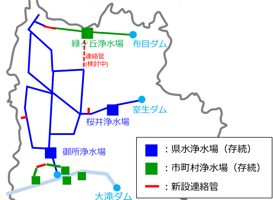
浄水場配置図（集約後）
