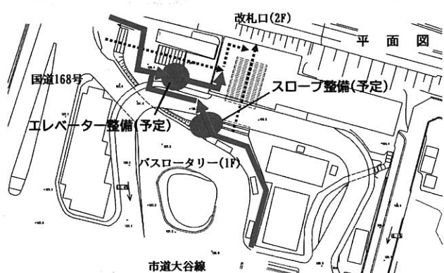
工事計画図(9月29日付生駒市HP報道資料から引用)
