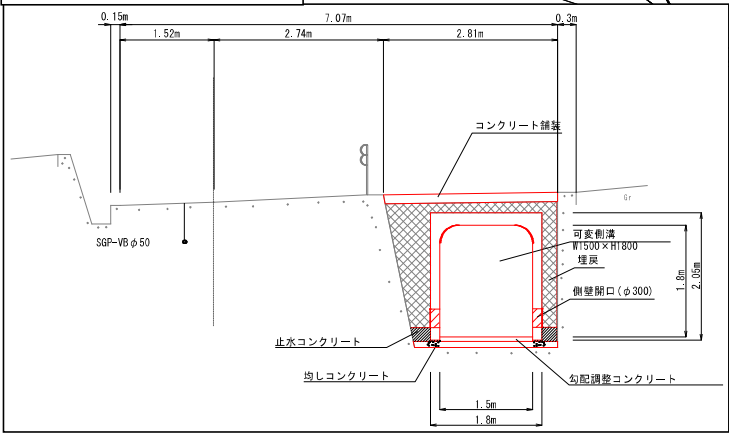
横断面図(案)
