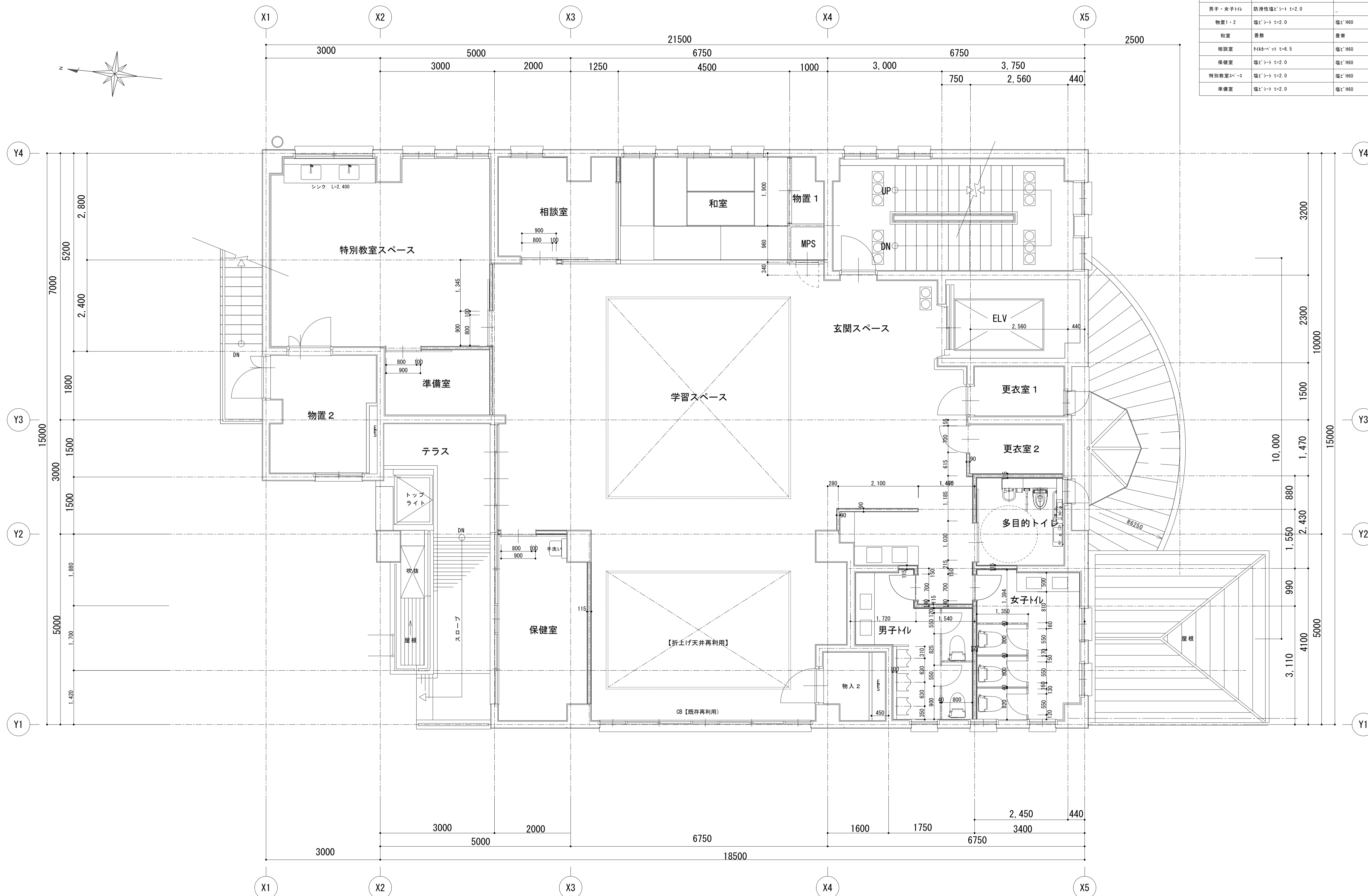
2階平面詳細図 1:50
