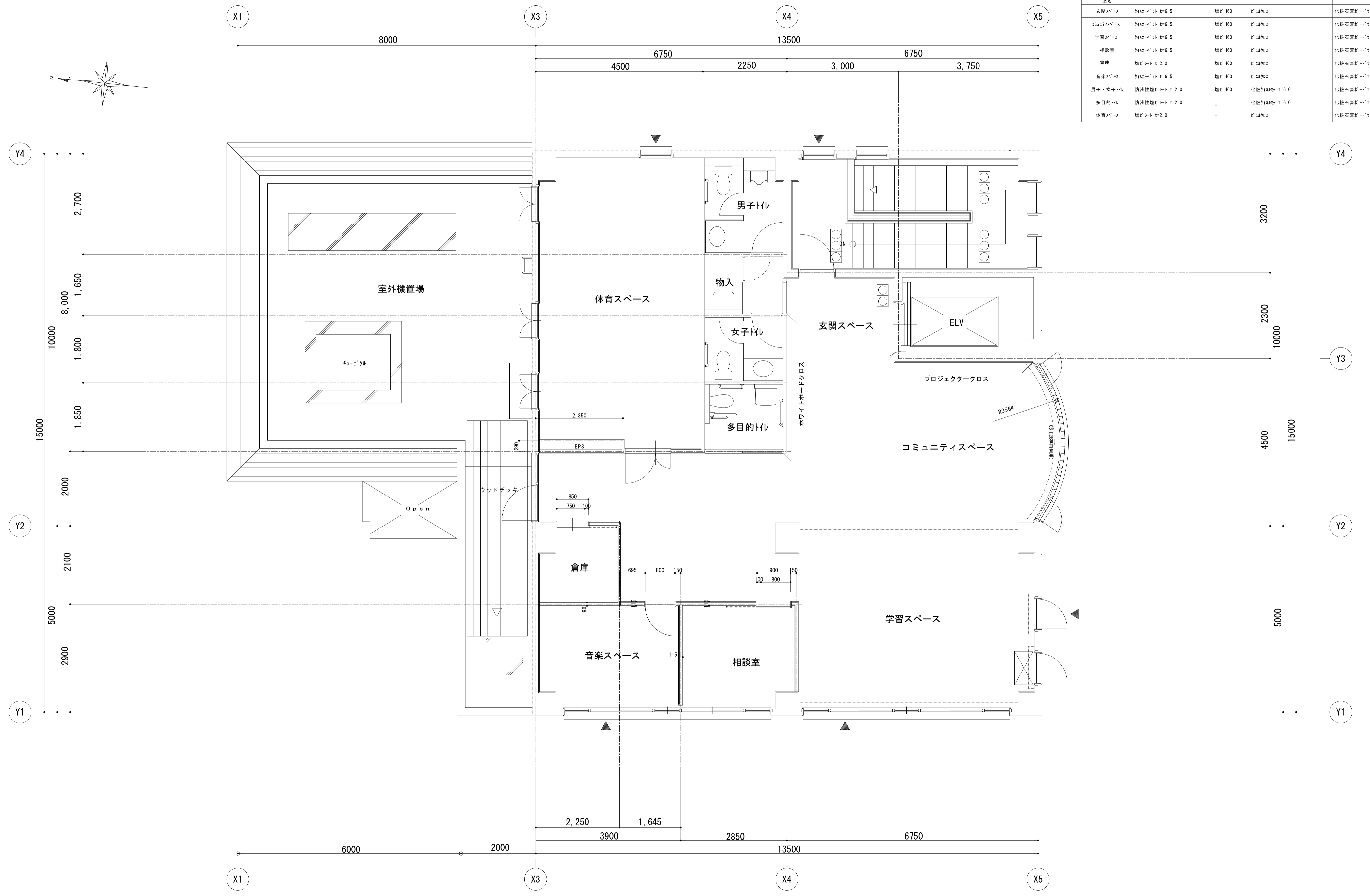
3階平面詳細図 1:50
