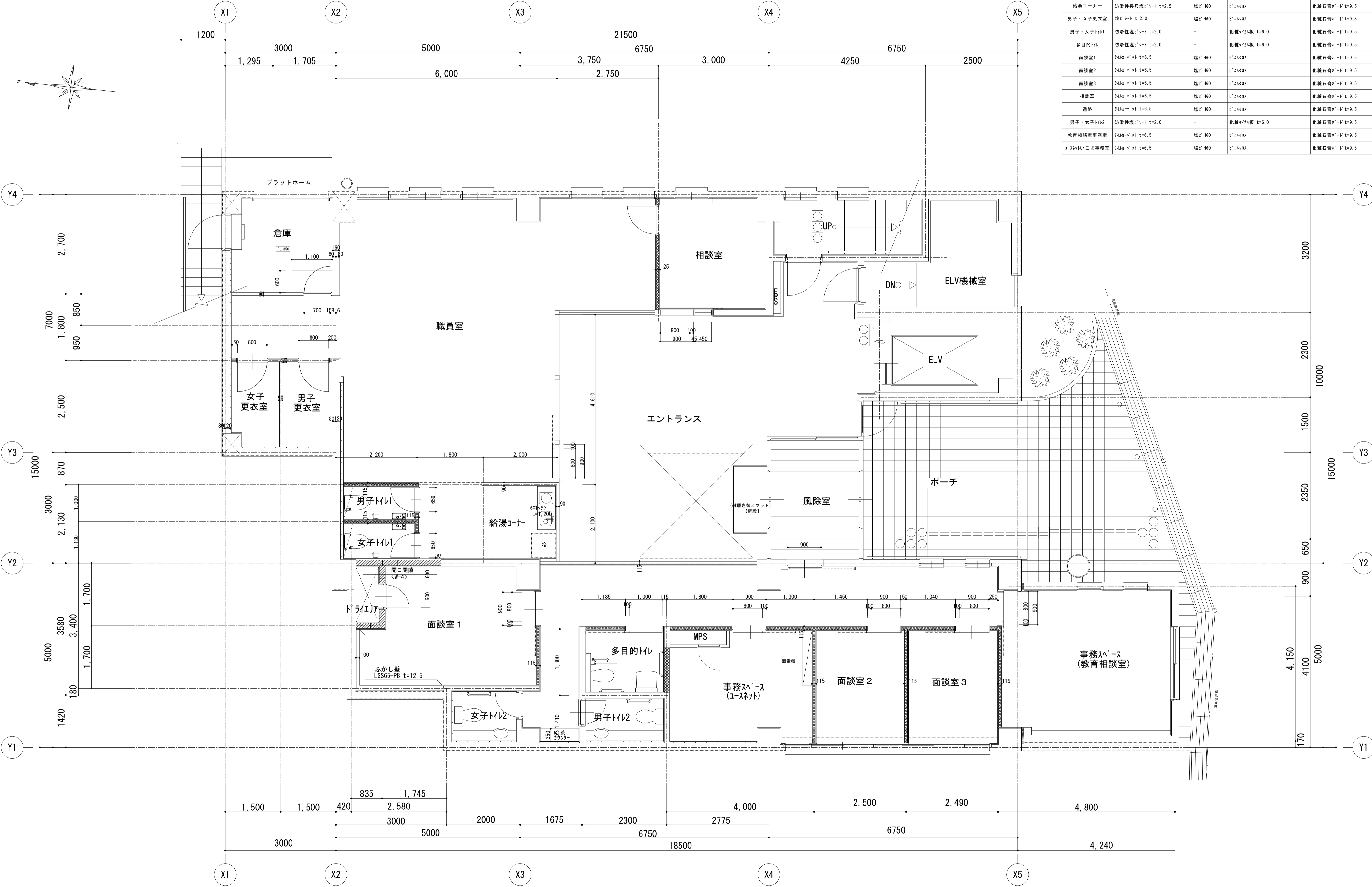
1階平面詳細図 1:50
