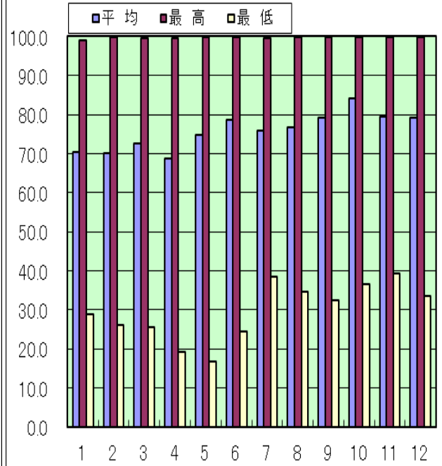
月別湿度(単位:%)
