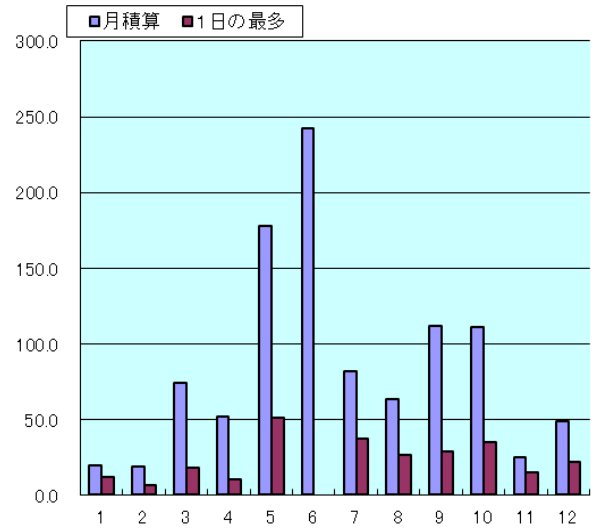
月別雨量(単位:mm)
