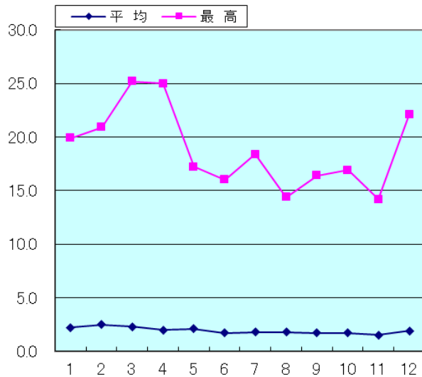
月別風速(単位:m/s)
