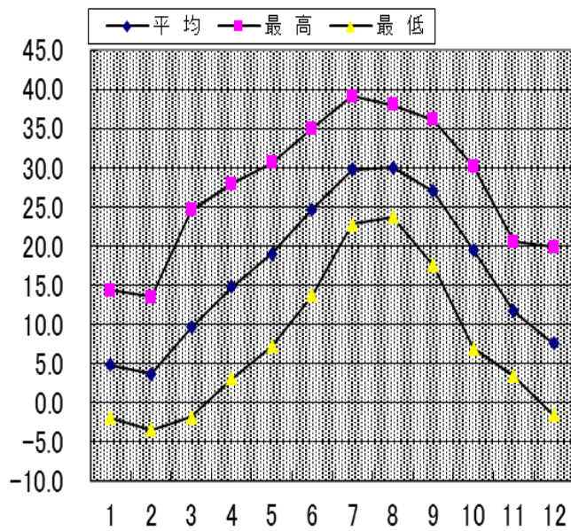
月別気温(単位:°C)
