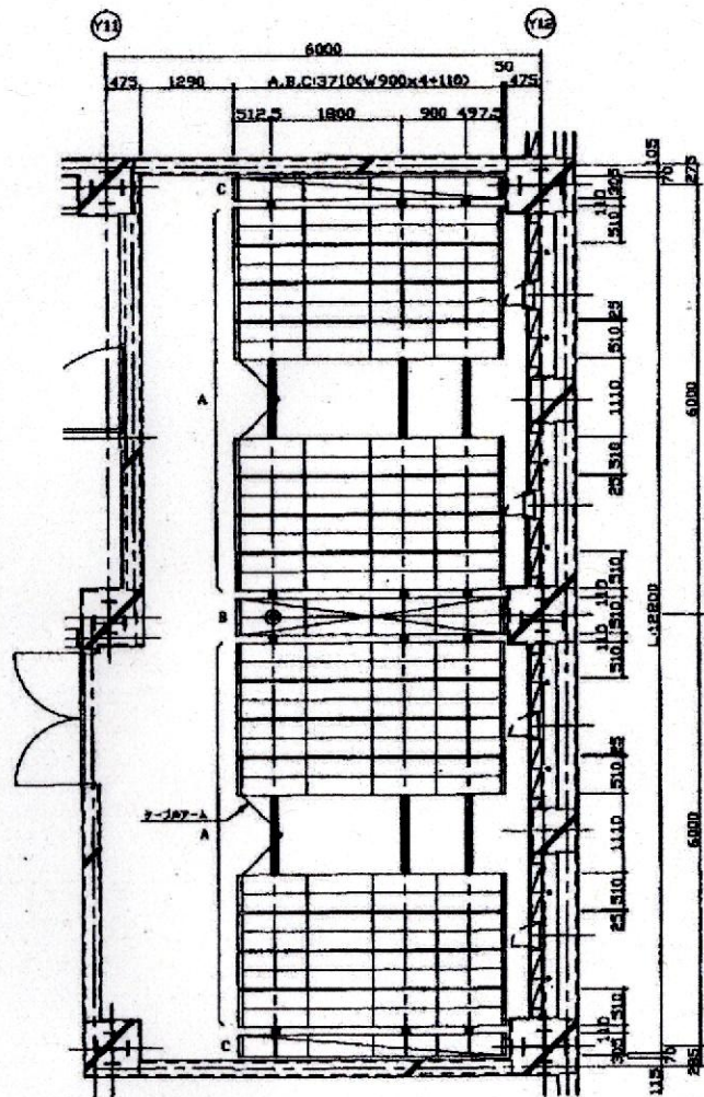
標準 設置図 S-1/50
