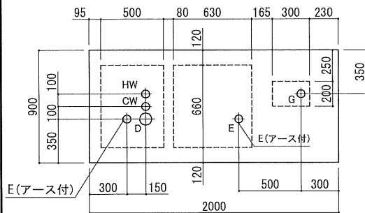
配管立上平面図 S1/30 (破線内は配管立上有効スペース)
