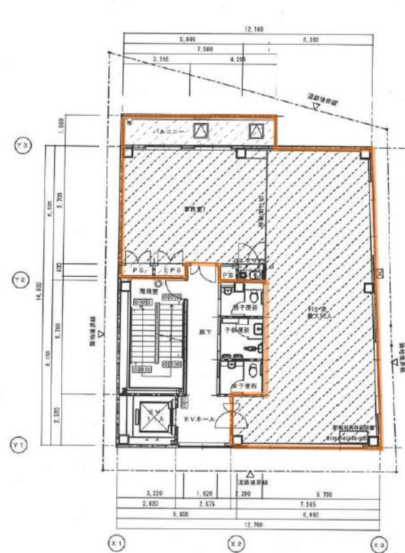
3階平面図(124㎡)
