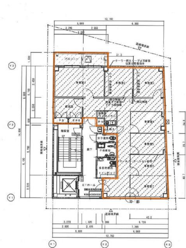
4階平面図(125㎡)
