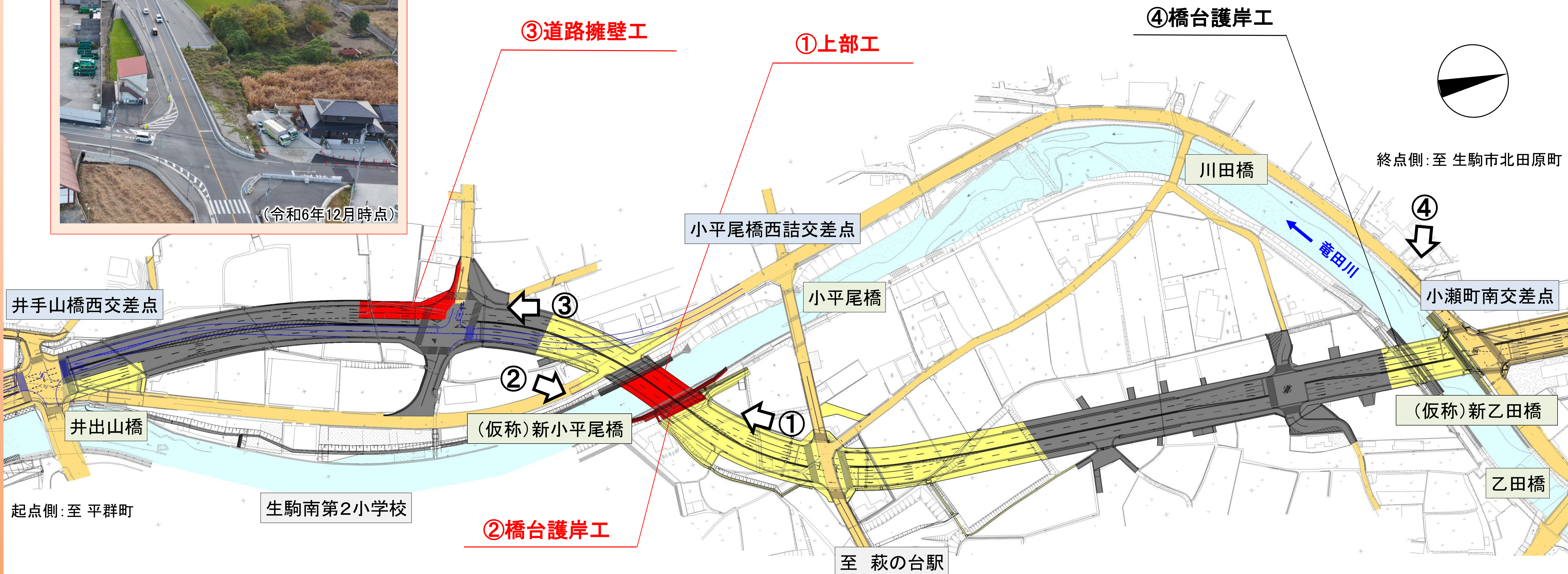
①(仮称)新小平尾橋 上部工
