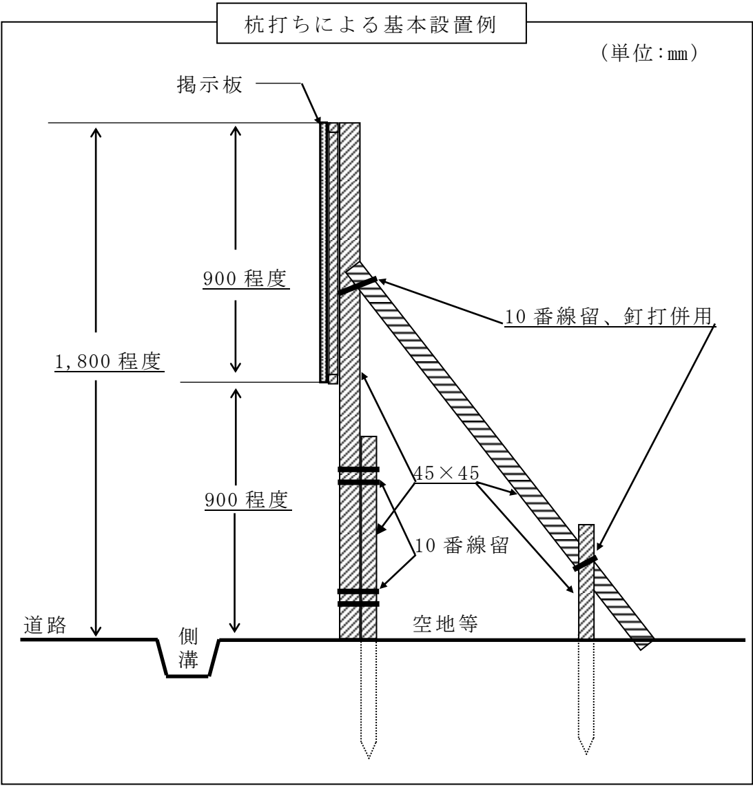
ポスター掲示場設置詳細図 No. 1
