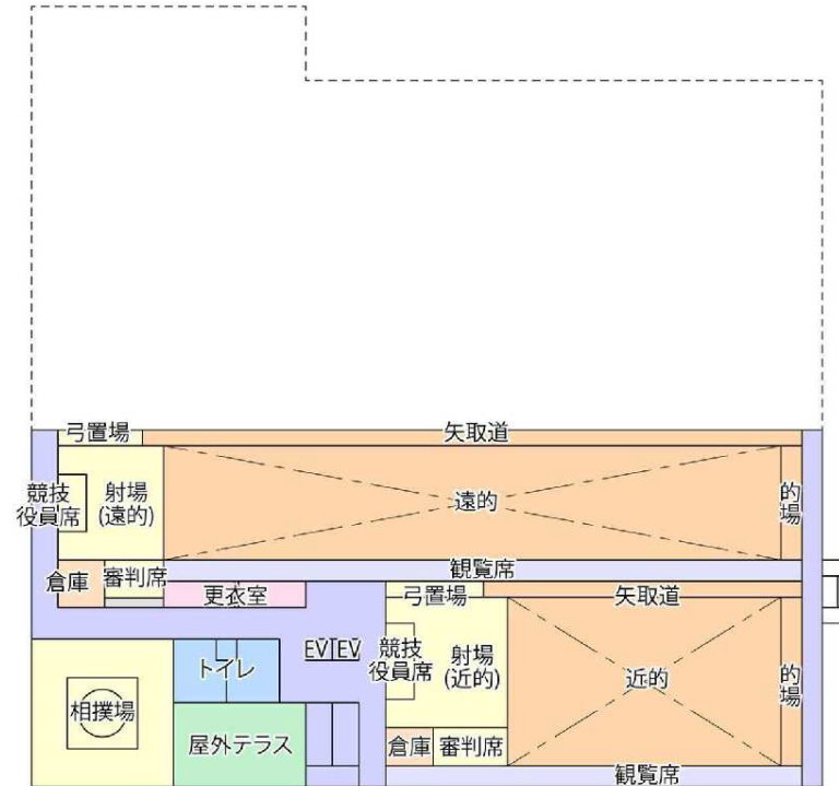
3階 平面図
