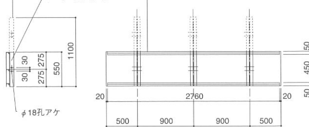
アルミ下地材 T-100×5×65×11 (一枚取付時)
