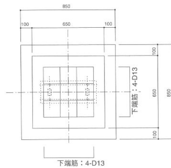
基礎図 1/20
