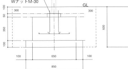
アンカーボルト M30-23 Wナット M-30
