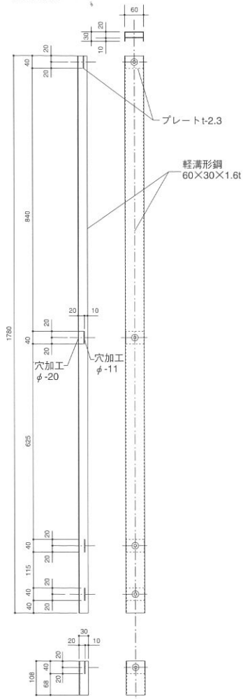
側板詳細図 1/10
