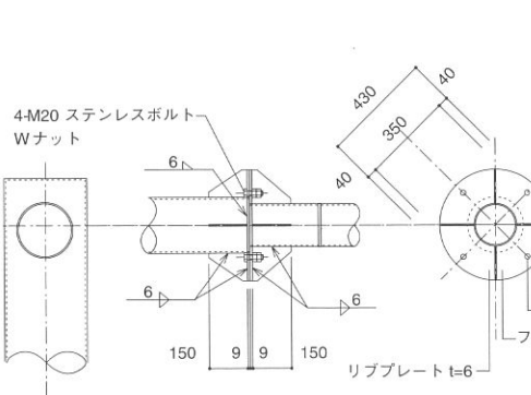
梁継ぎ部 1/40
