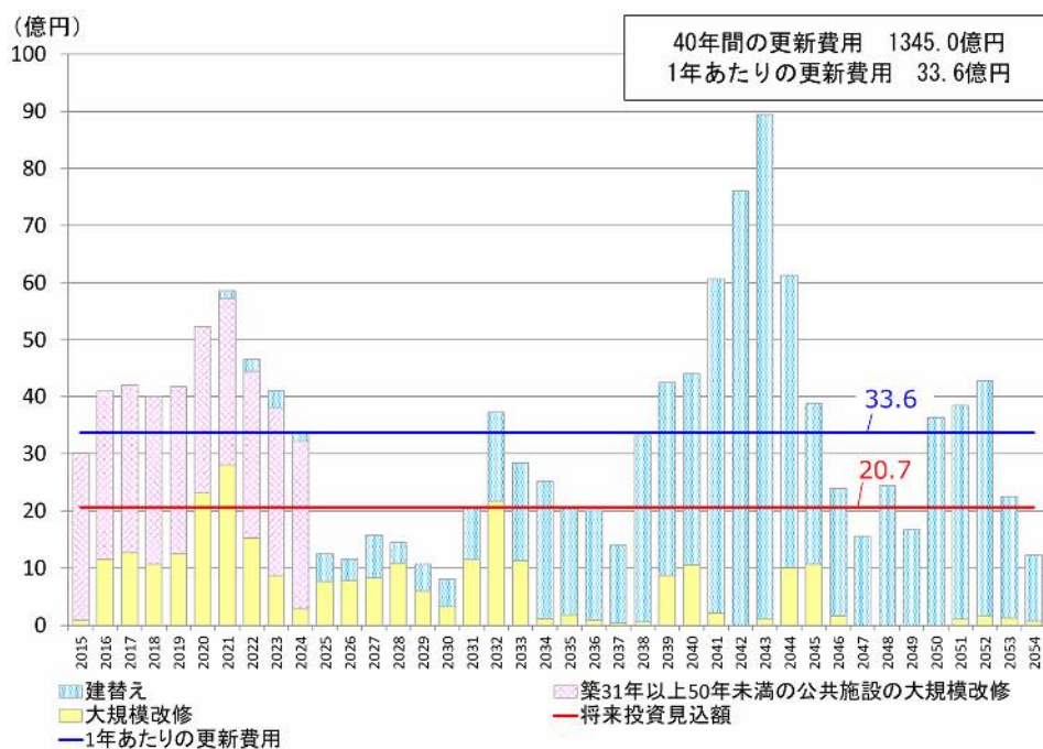
図 インフラ施設の将来の更新費用の推計
