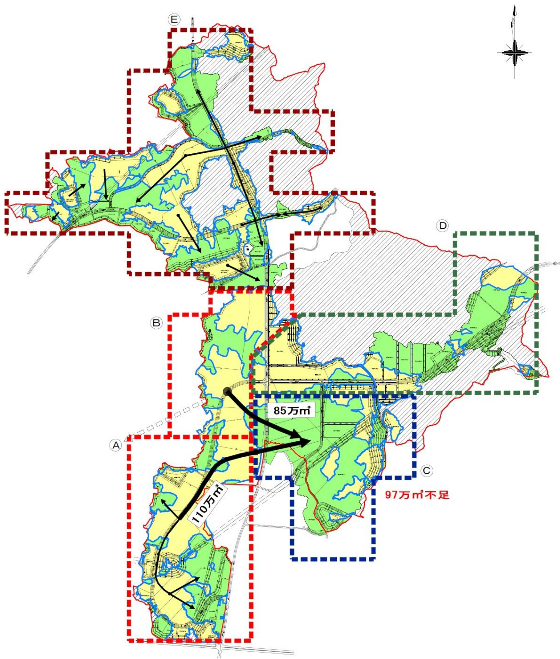
H21年度高山地区第2工区運土計画図
