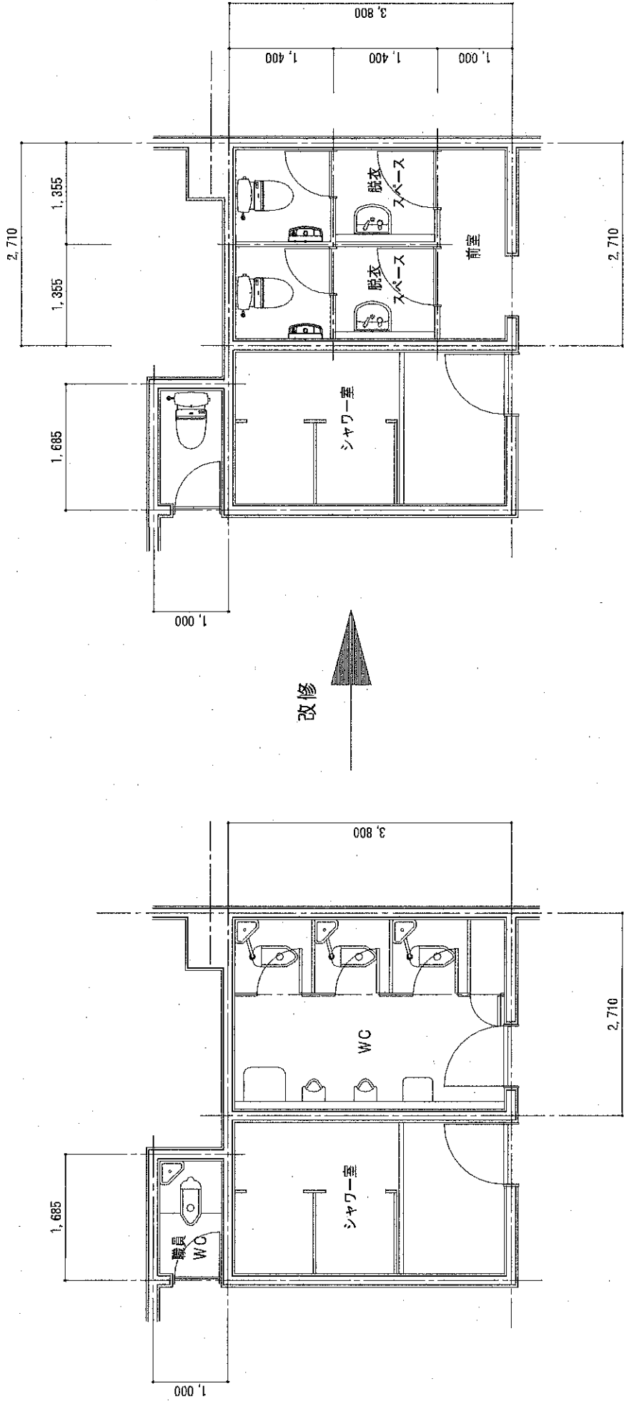
現況平面図
