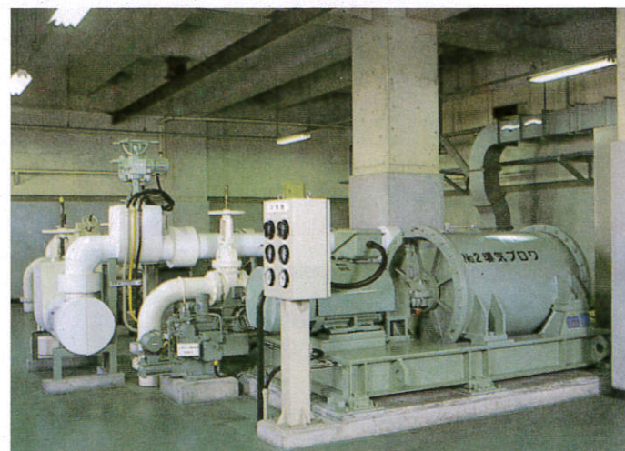
曝気ブロー
