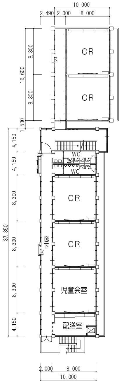
3階 平面図
