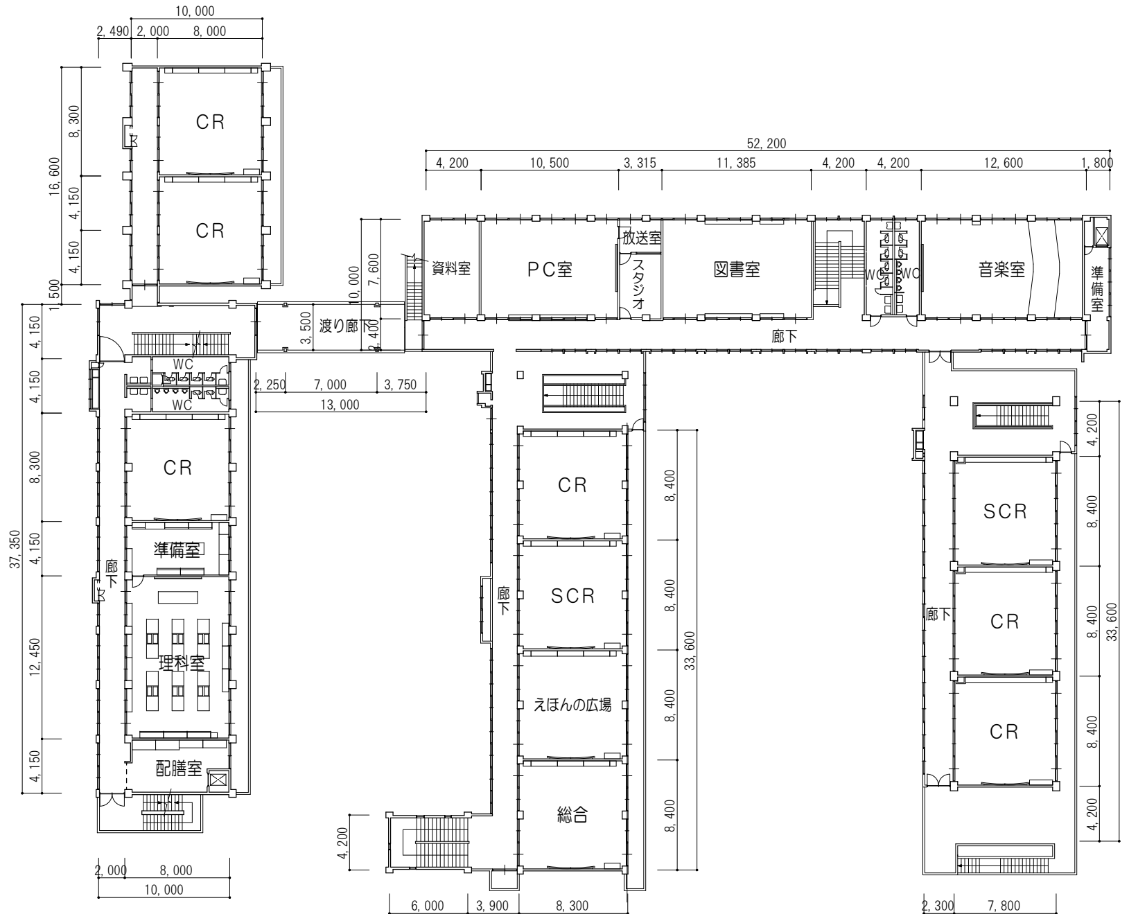
2階 平面図
