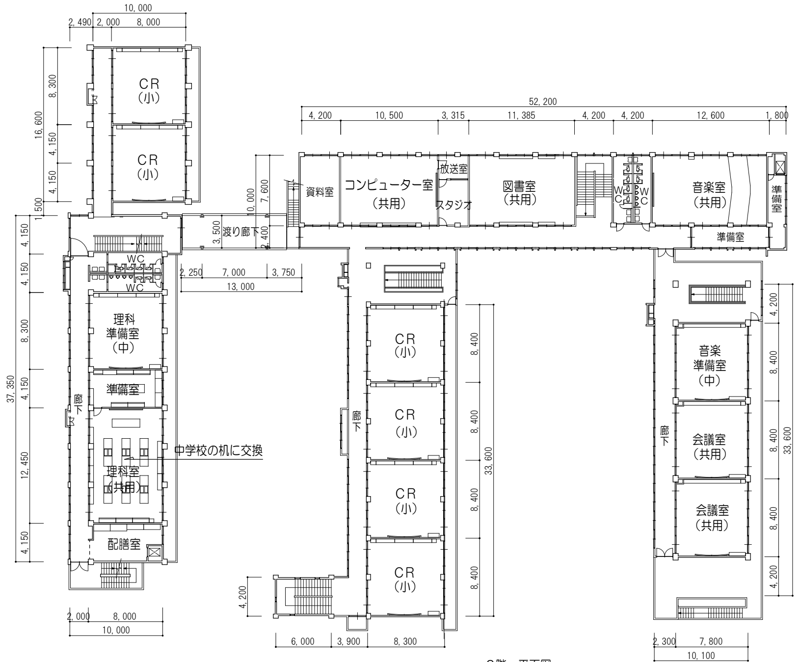
2階 平面図
