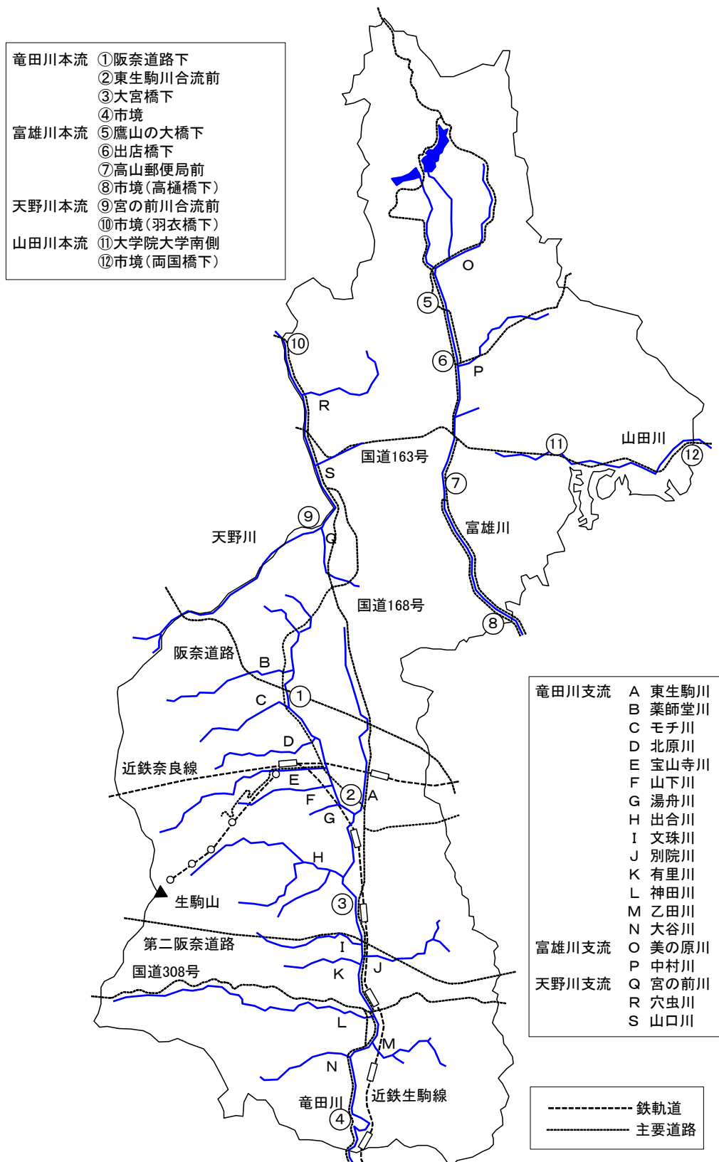
図表 79 河川水質測定地点
