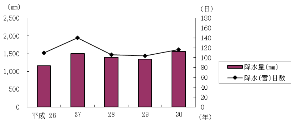
図表 8 降水量及び降水(雪)日数
