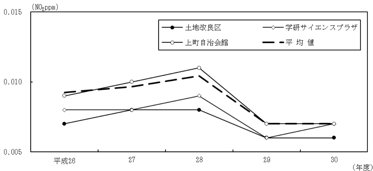
図表 67 二酸化窒素濃度測定値（北地区）
