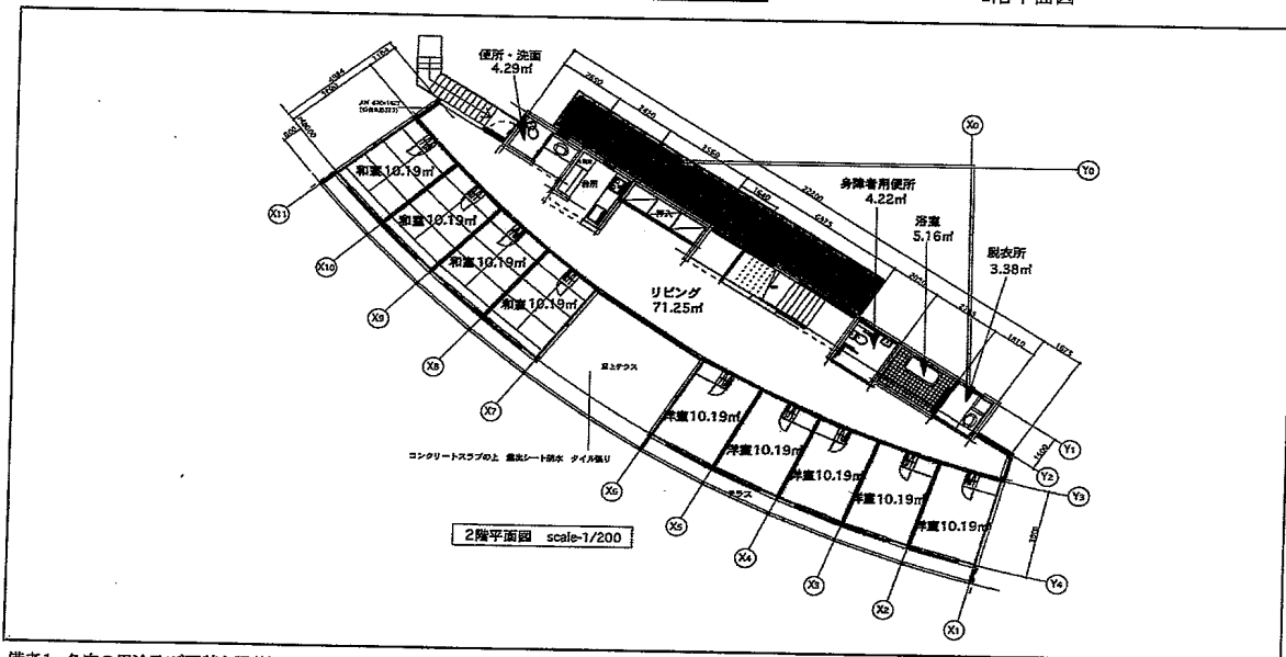
2階平面図
