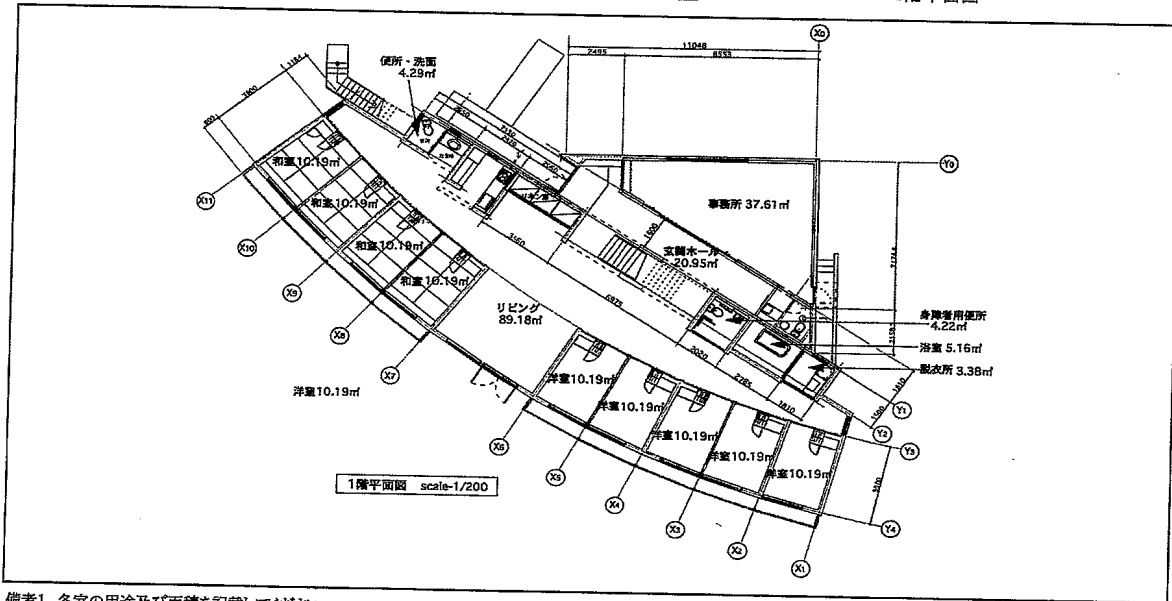
1階平面図
