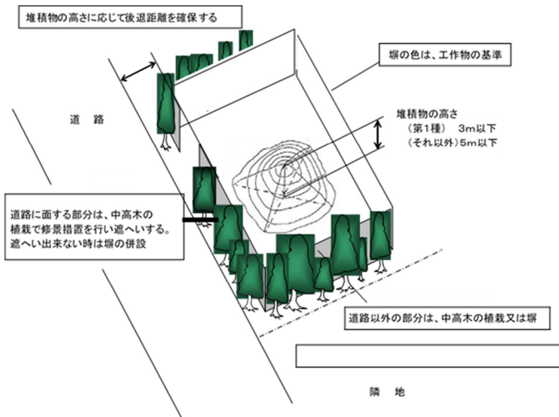
[図1] 資材置き場の植栽等基準モデル
